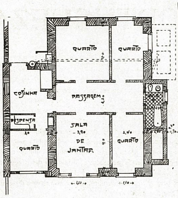
12,50 Planta do rez-do-chão
