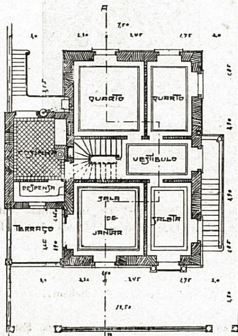
11,75 Planta do 1.º andar
