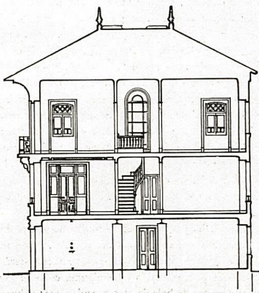
Corte A B
