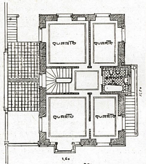
7,50 11,50 Planta do 2.º andar
